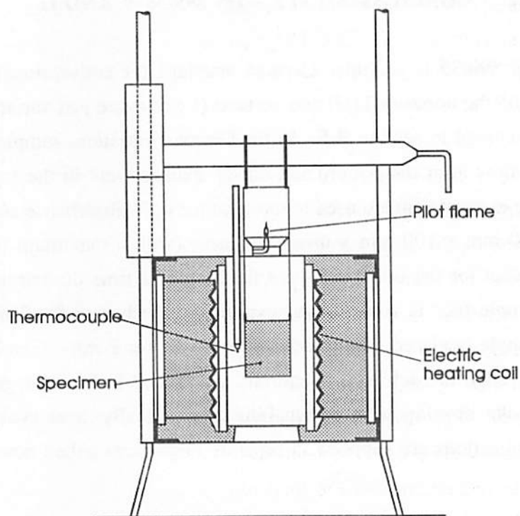
Figure D2. The DIN 4102 Furnace Test
