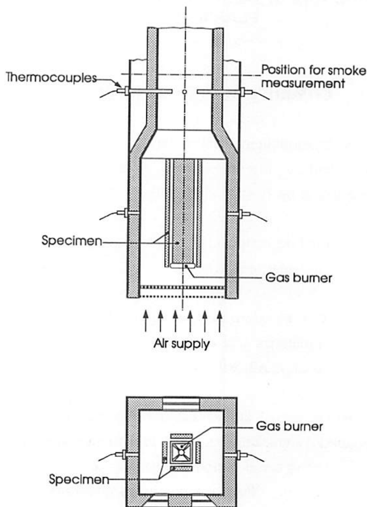
Figure D1. The DIN 4102 Fire Shaft or “Brandschacht” test
